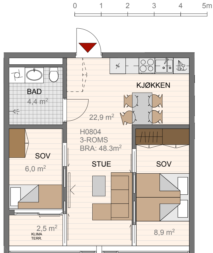
Leil Type 5s (3 roms speilvendt)
